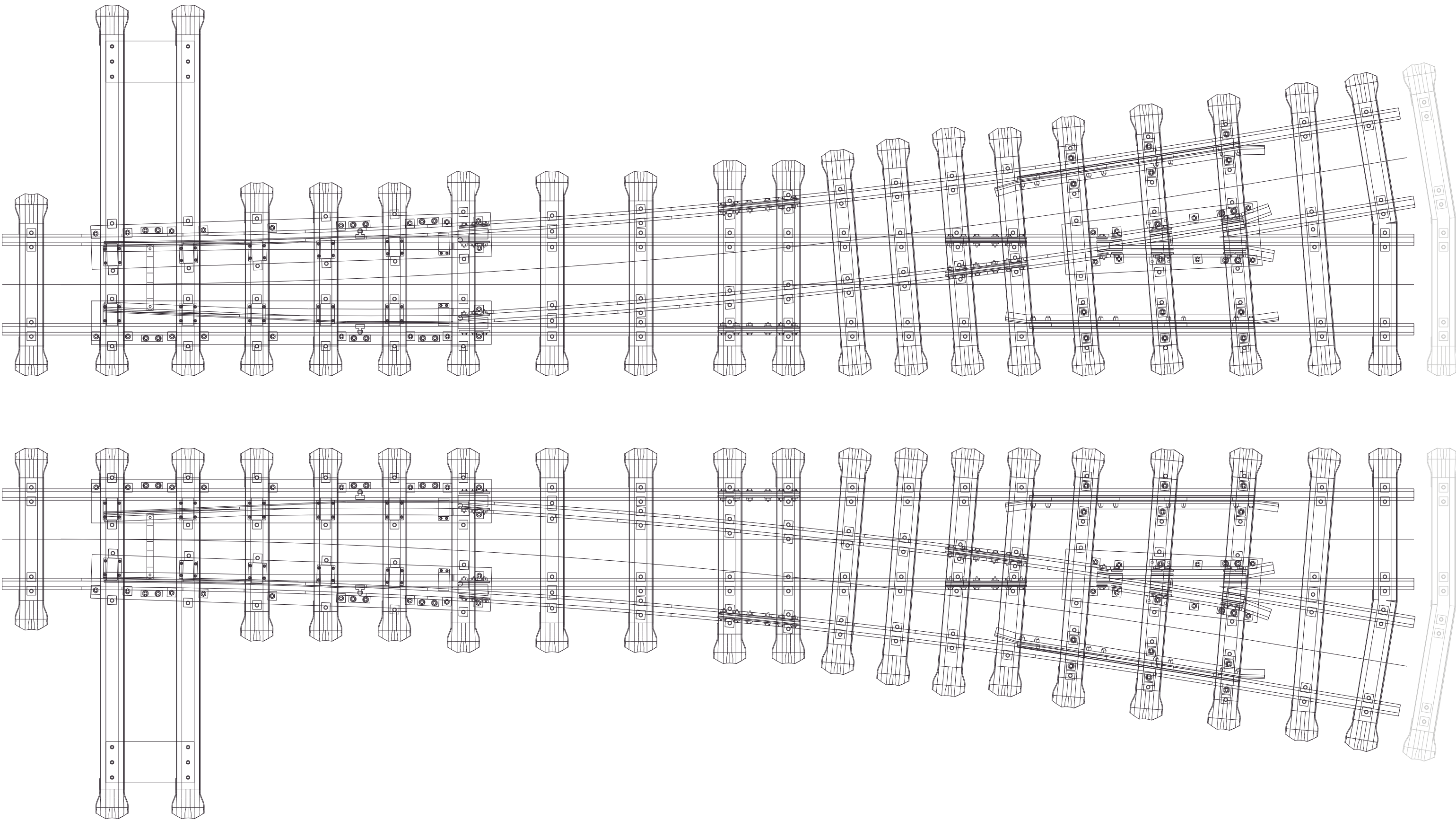
Planungsbogen 1:1 Spur 1e (23.4 mm) Einfache Weiche der DRG D-70-1:6 (RBD Stuttgart), Württemberg Copyright © 2016 WENZ-MODELLBAU
