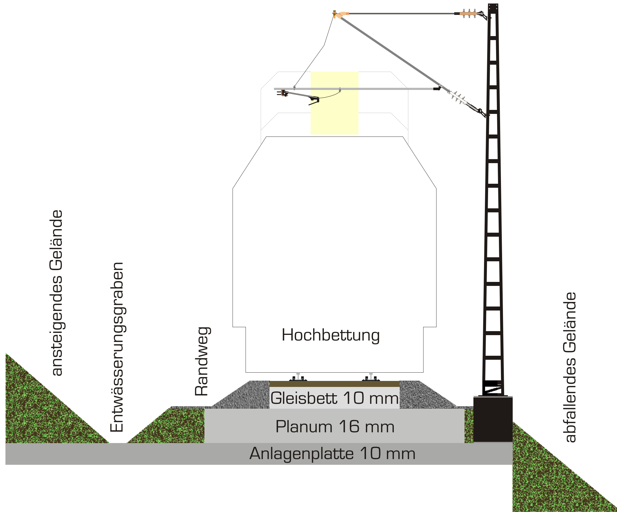
Vorbildgerechter eingleisiger Bahnkörper Deutsche Bundesbahn Maßstab 1:1 für Spur 0 Copyright © 2008 WENZ-MODDELLBAU - Alle Rechte vorbehalten.
